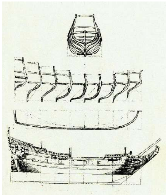
Рис. 10. Конструктивный чертеж пинасы середины XVII в. (по: Генриот, 1974, с. 167, рис. П. 46).
